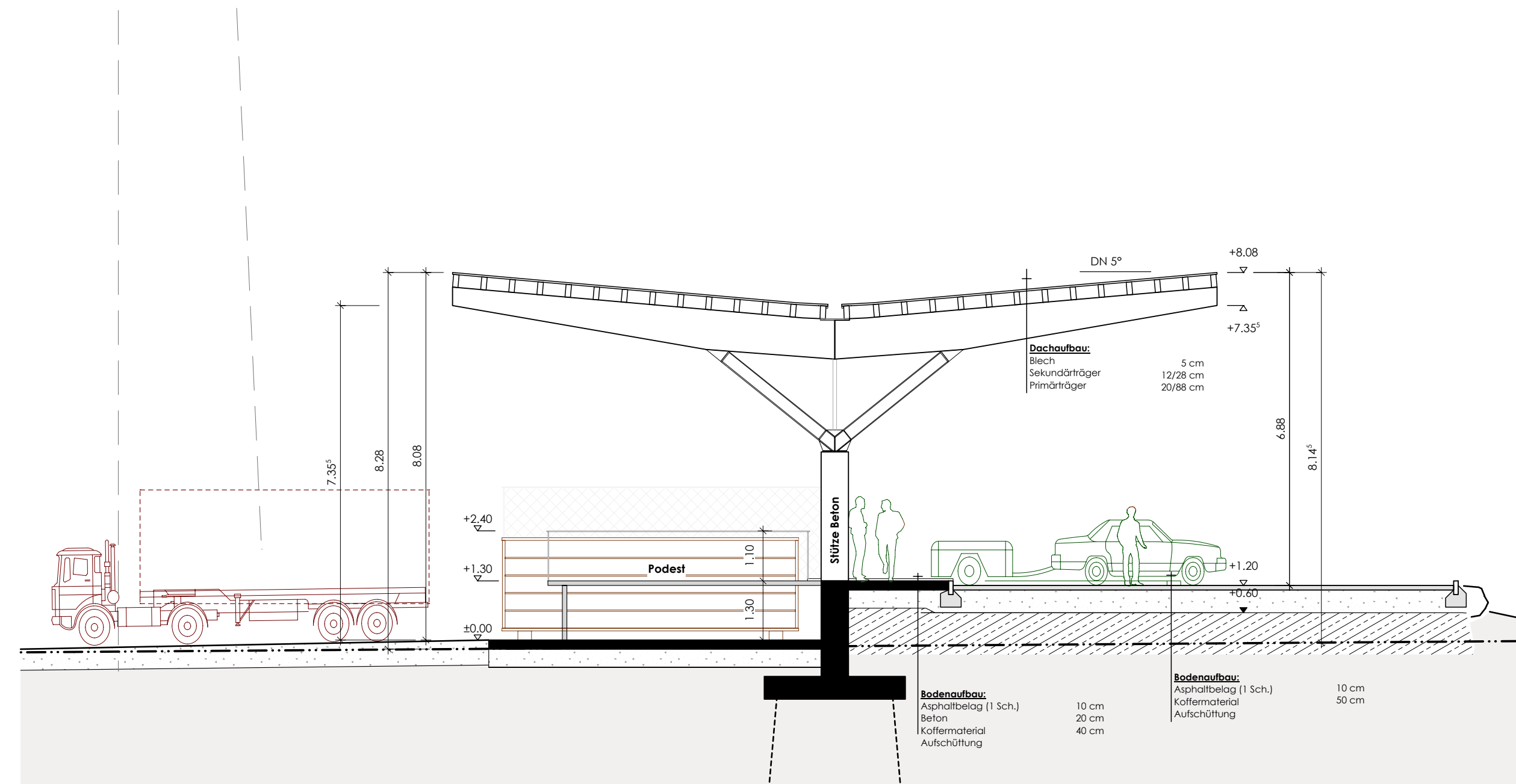
Querschnitt
